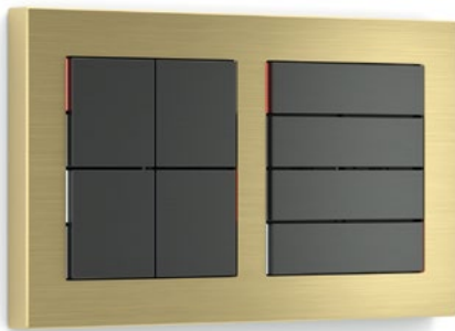
E12 – 4tlačítkový vypínač s měřením teploty – dvojnásobný rámeček. Rámeček i hmatníky jsou v provedení: broušený kov – mosaz a karbon, červená/bílá LED. Rozměry: 87 x 158 x 9 mm.
