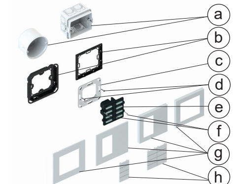
Montaggio per scatola quadrata o rotonda
