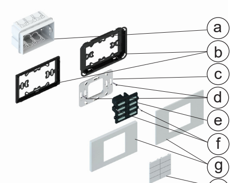
Montaggio per scatola rettangolare
